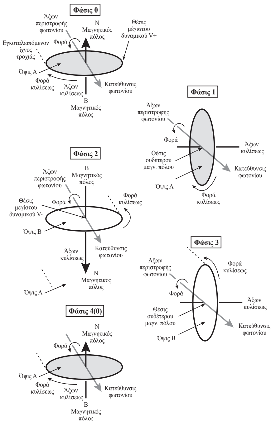
Σχηματική παράστασις περιστροφής και κυλίσεως φωτονίου και εναλλαγών δυναμικού
