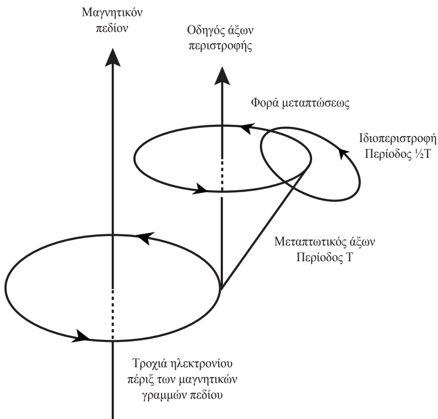
Σχηματική παράστασις κλασματικού σπιν ηλεκτρονίων
